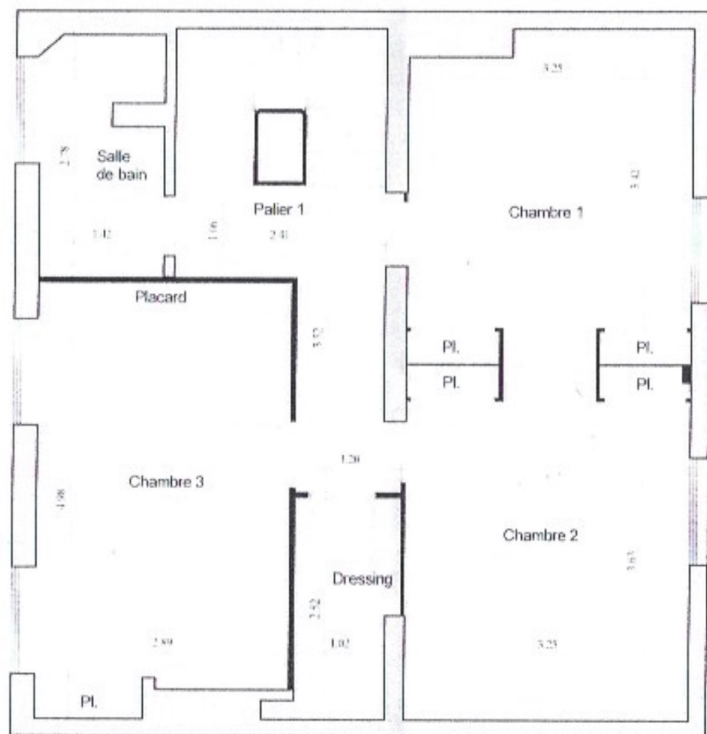
1 er étage
