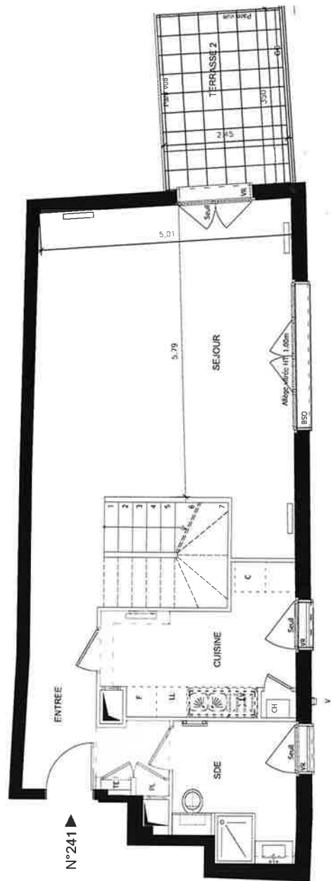
4 ème ETAGE
