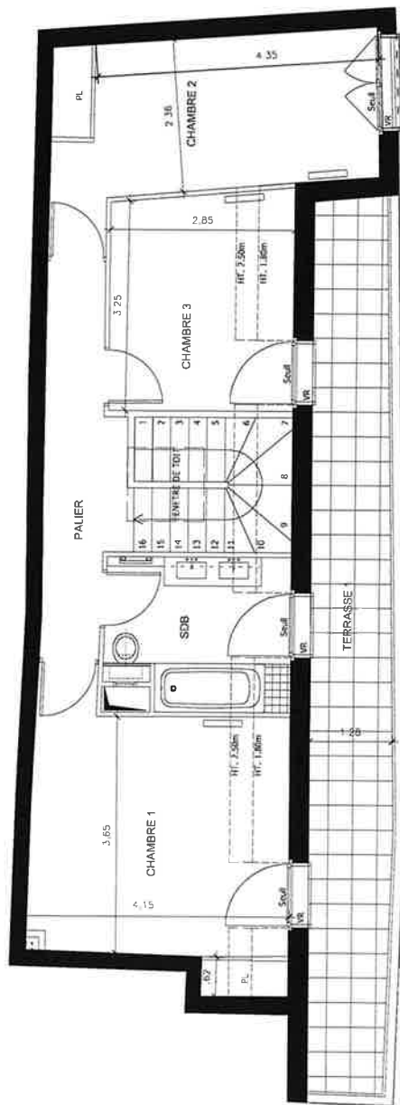
5 ème ETAGE
